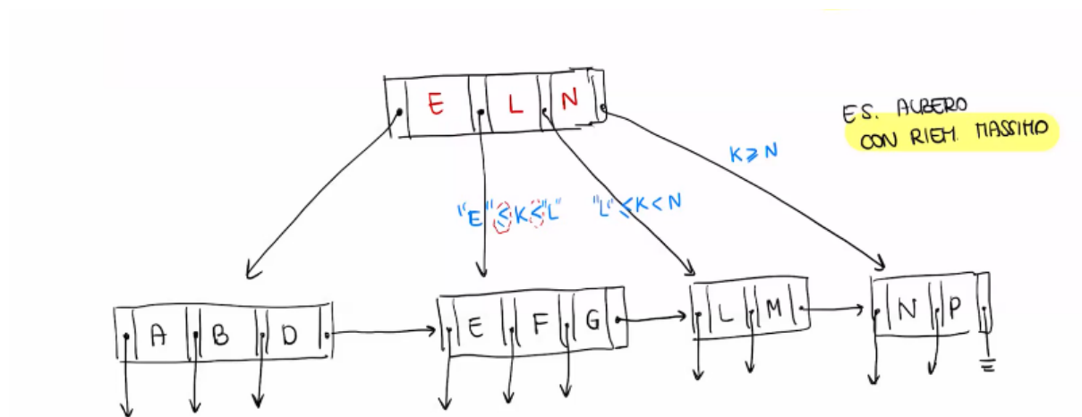
Figura 114: Esempio 1 : Albero con Riempimento massimo
