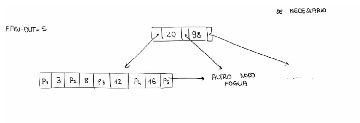
Figura 119: Stato iniziale: fan-out n = 5 , nodo foglia contenente i valori 3, 8, 12, 16
